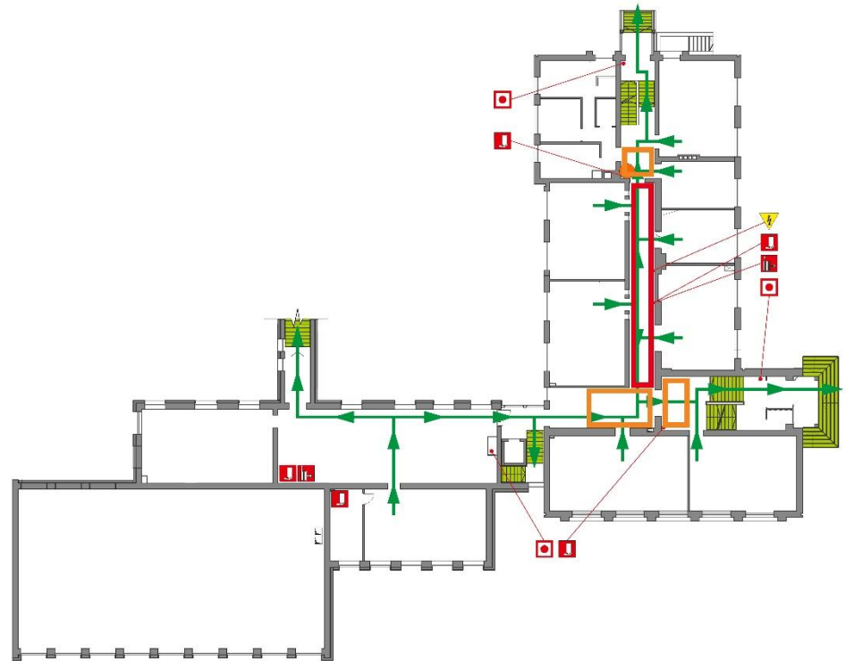
1.stāvs
